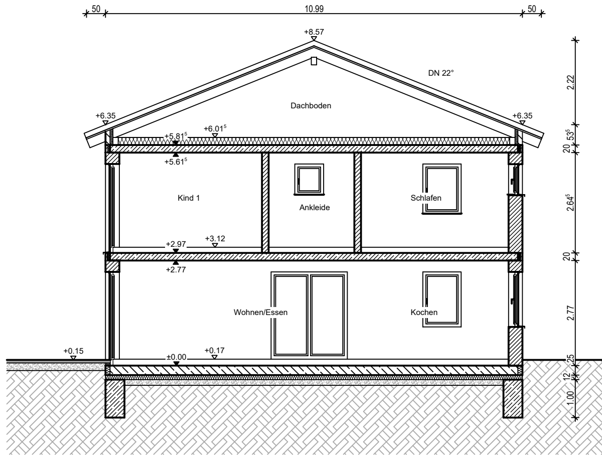
Schnitt A-A
